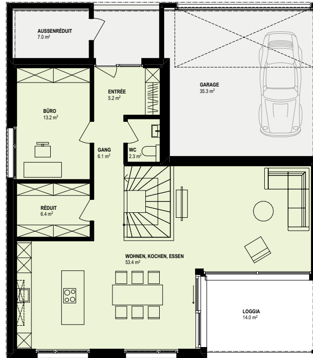
Grundriss Obergeschoss
